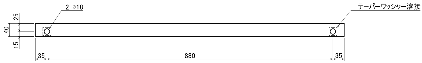
盤固定金具 (溝型鋼 75×40×5×7)
